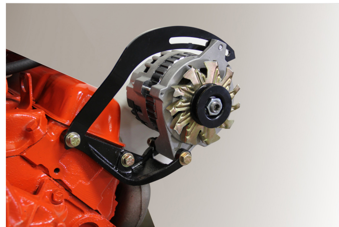
6772ABK_install.jpg
