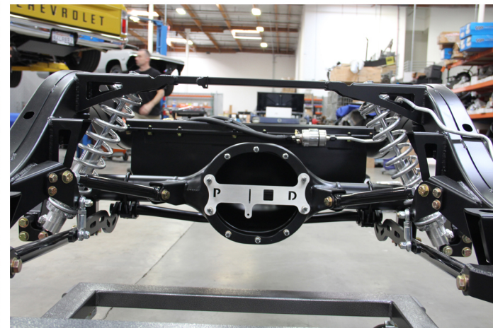
5557RFL-K_REAR 4 LINK_install_1.jpg
